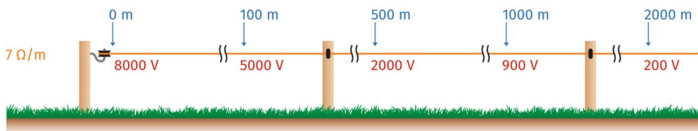
Scăderea de tensiune într-un gard electric construit cu fir de 7 \Omega/m
