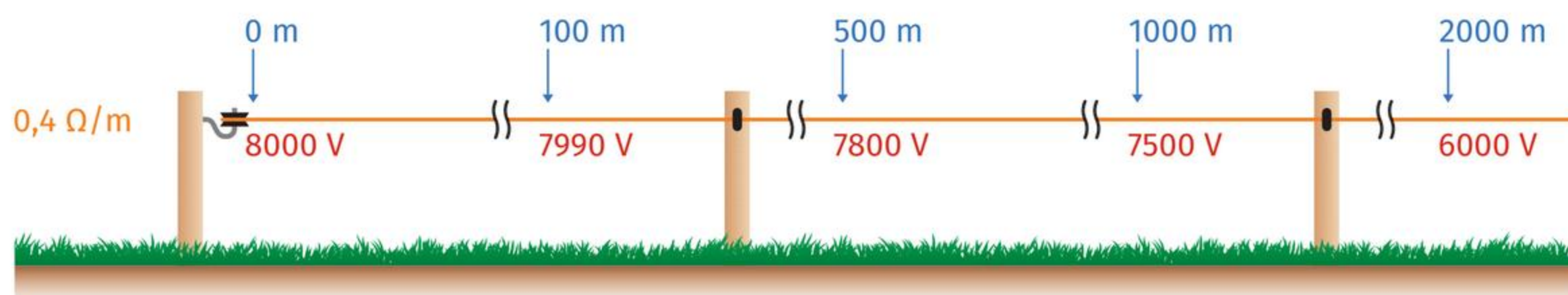
Scăderea de tensiune într-un gard electric construit cu fir de 0,4 \Omega/m
