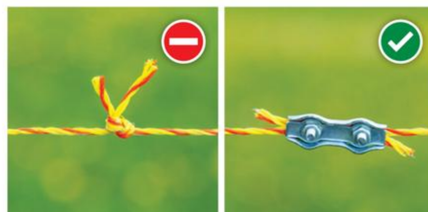
Nu folosiți noduri pentru prelungirea firului!
